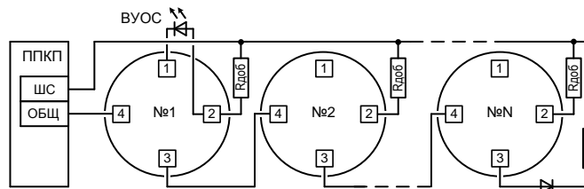
Рис.2 Типовая схема подключения извещателей к ППКП со знакопеременным ШС. Величина резисторов R_{ок} и R_{доб} определяется в соответствии с техническим описанием ППКП.
