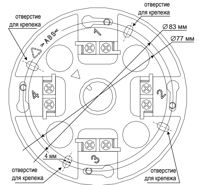
Рис.4 Базовое основание извещателя. Расположение отверстий для крепежа.
