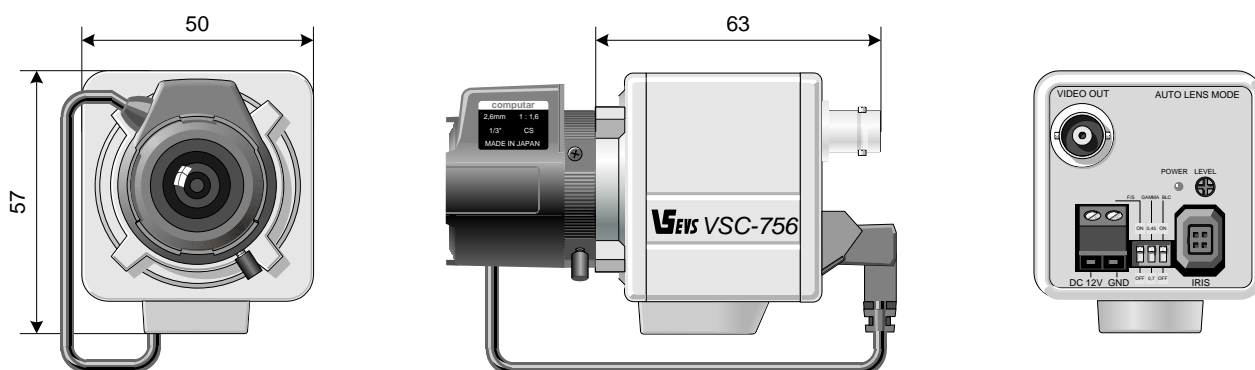
Рис.2. Камера VSC-756
