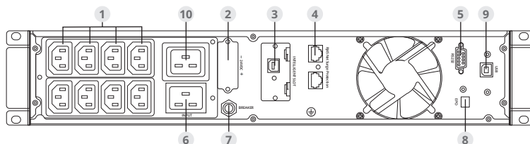
Вид сзади: ИБП ИМПУЛЬС ФРИСТАЙЛ 3000 ВА
