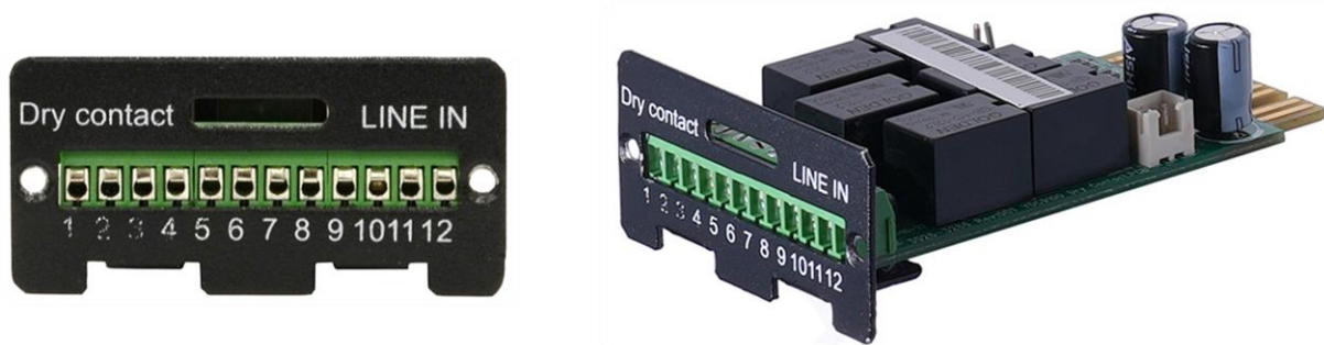
Внешний вид карты релейного интерфейса
