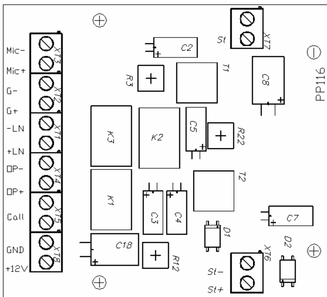
Рис. 2 Вид платы PE113 блока сопряжения.
