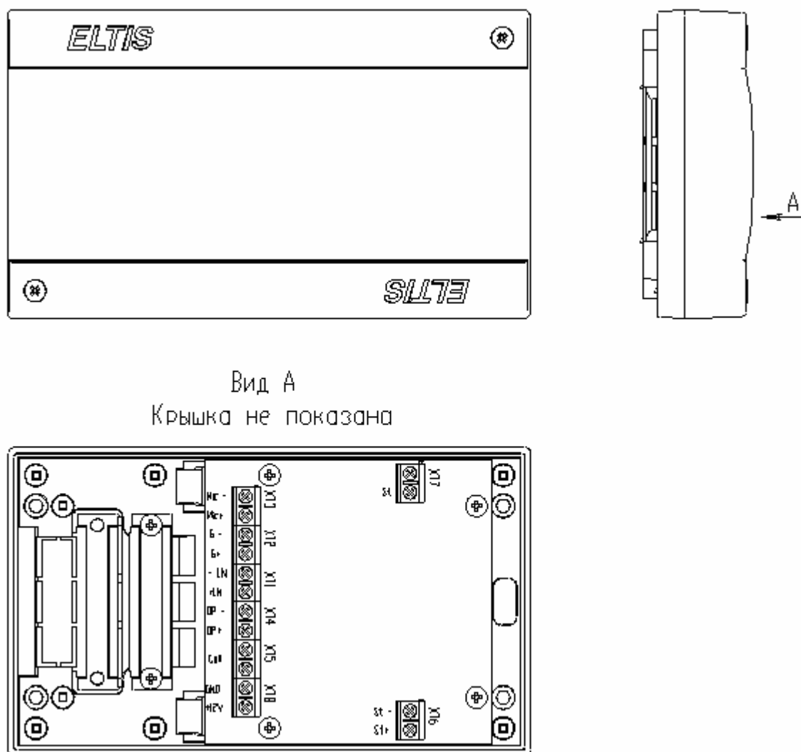
Рис. 1 Внешний вид блока сопряжения
