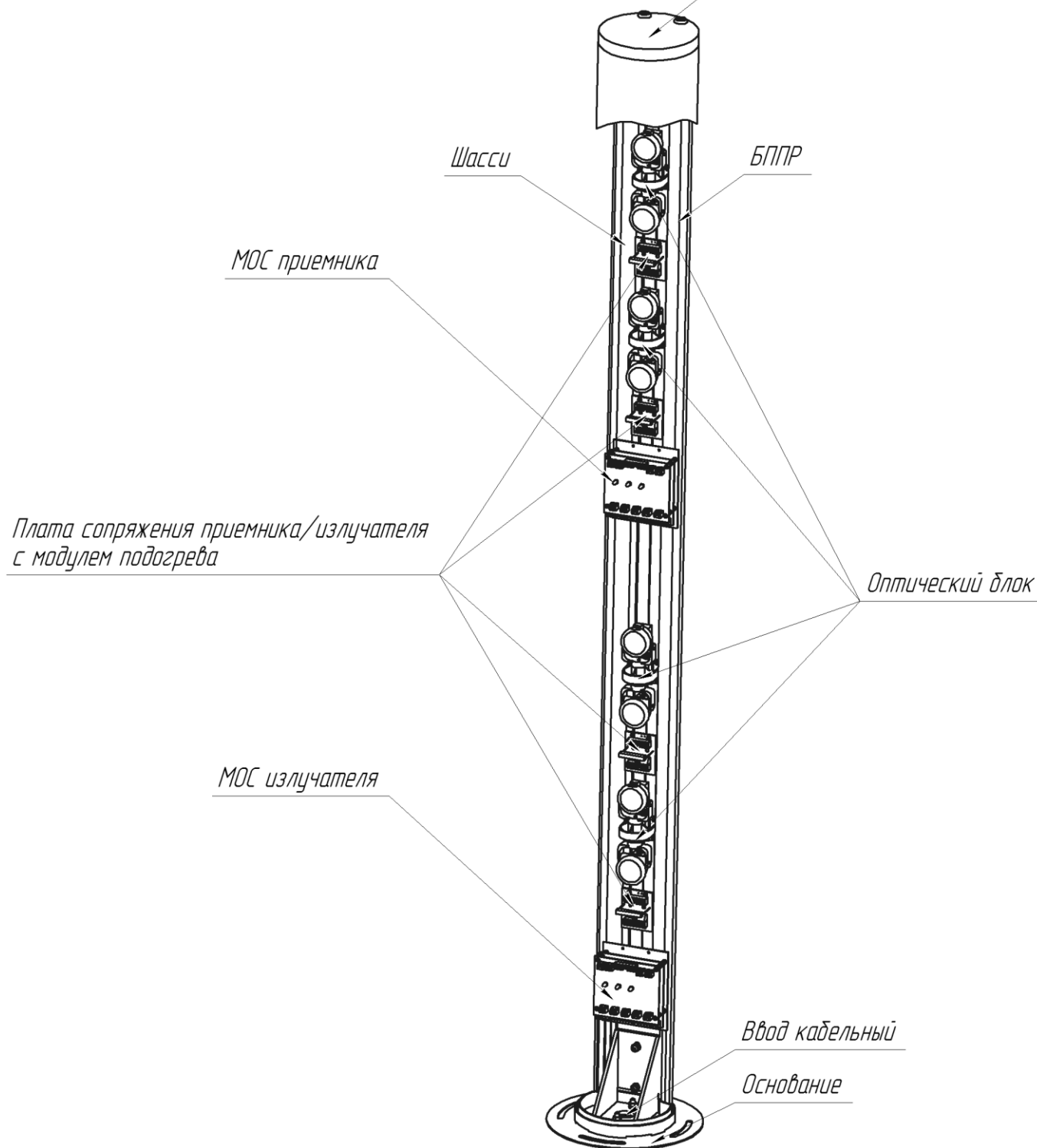
Рисунок 1.4 – Внешний вид БППР изделия «ПАНТЕРА-2»
