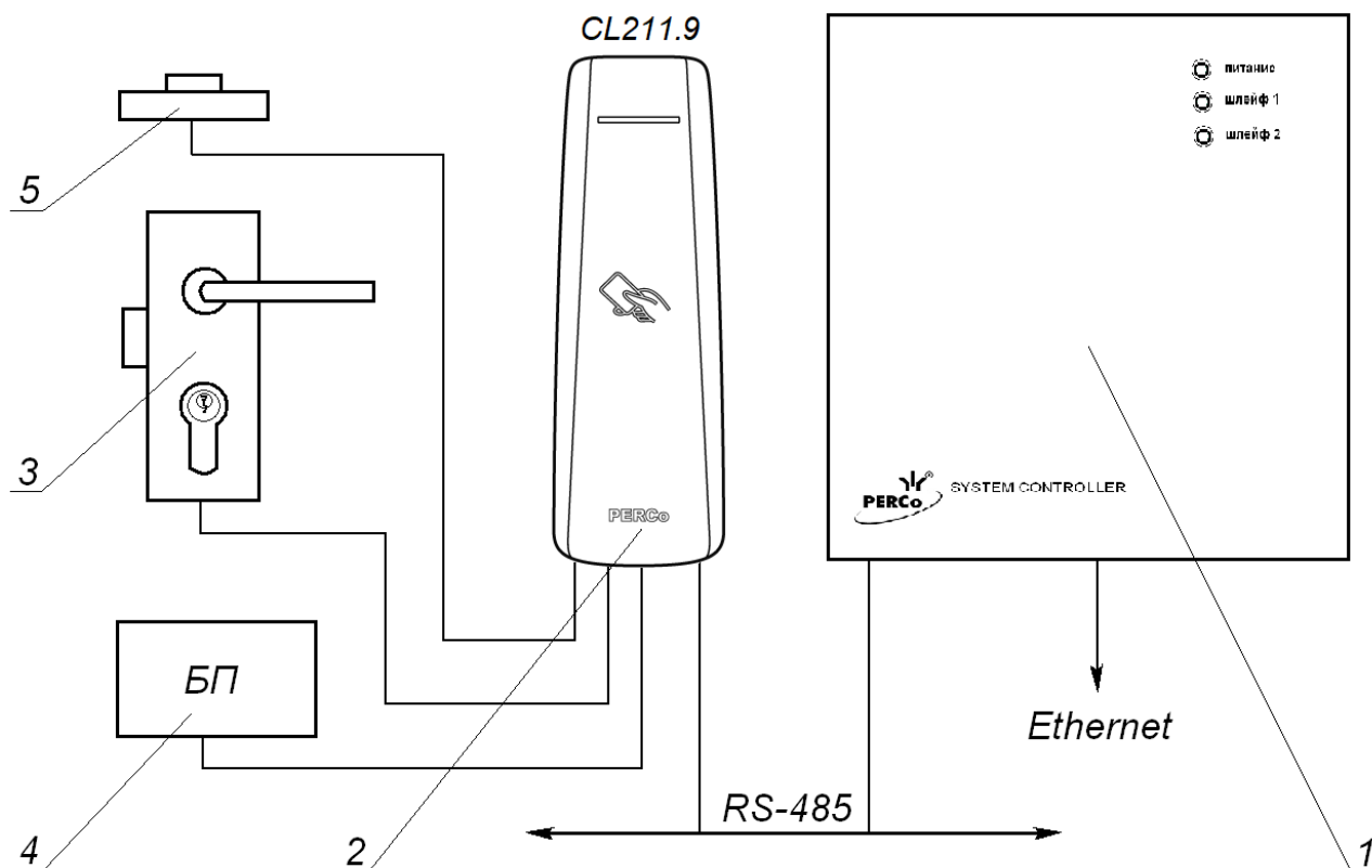
Рисунок 1. Функциональная схема
