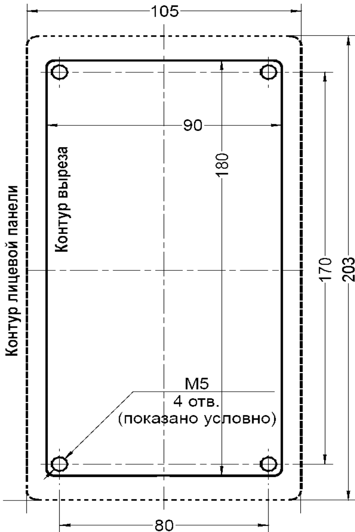
Рис. 1 Разметка под установку блока вызова
