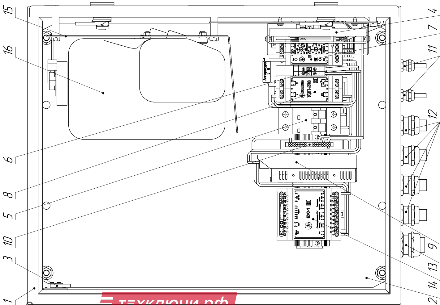
Рис. 1. Устройство термошкафа (дверь открыта на 90°)
