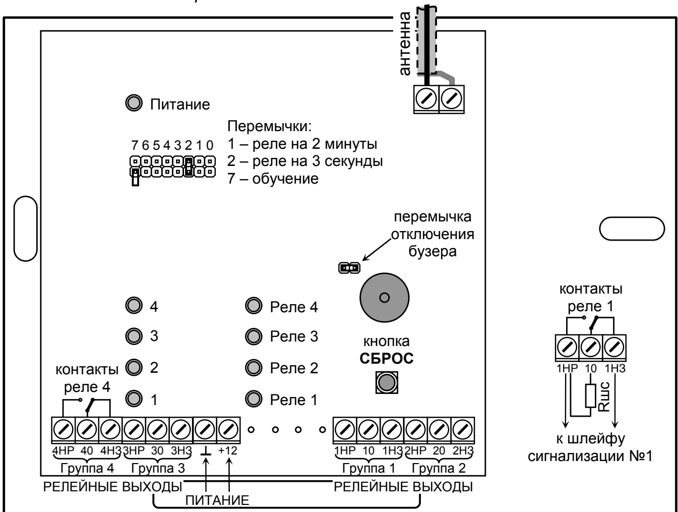
Рис. 2. Монтажная схема приемника и пример монтажа реле в шлейф
