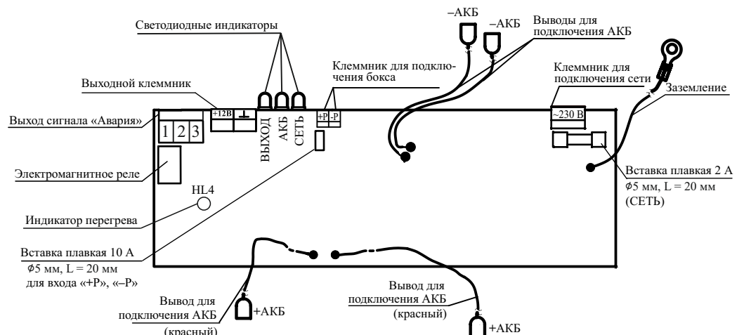
Рисунок 1 – Плата источника
