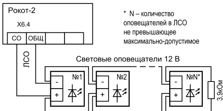
Рис.А5 Схема подключения световых оповещателей к ЛСО
