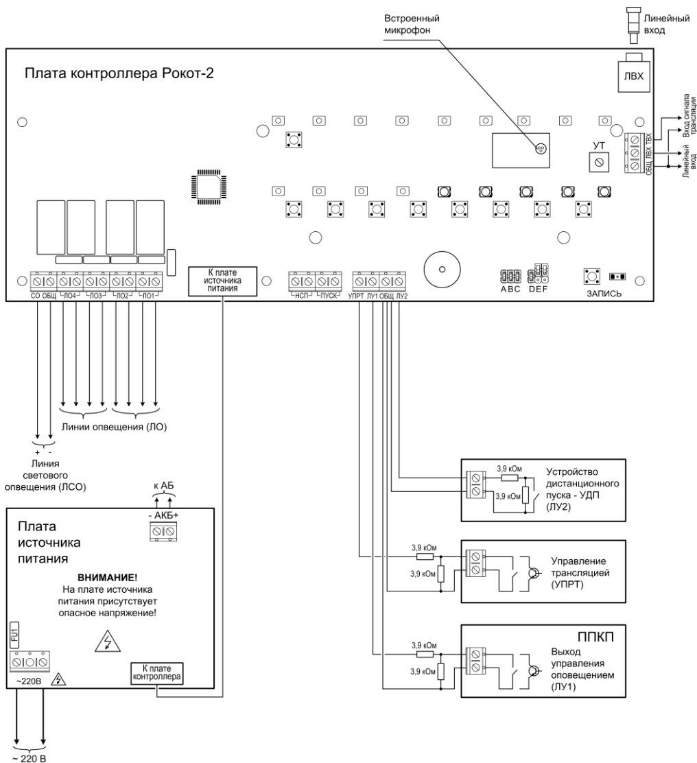
Рис.А1 Плата контроллера (вид со снятой панелью индикации и управления), плата источника питания и схемы внешних подключений прибора
