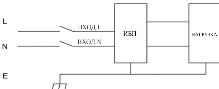
Схема соединения на входе — «однофазная с заземлением».
